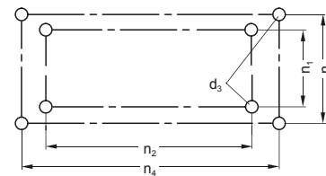
Montagelochung Footprint
