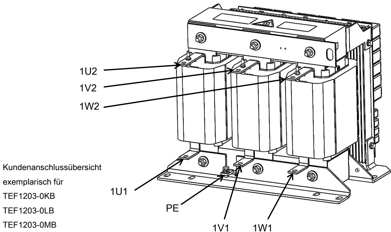
Bild 4-4 Kundenanschluss du/dt-Filter TEF1203-0KB
