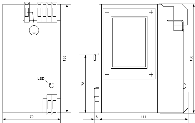
Schnappbefestigung auf Tragschiene / Snap-on fastening on DIN rail Bild 03 / Fig. 03: Raumbedarfsmaße und Anschlüsse / Space requirement dimensions of Terminals
